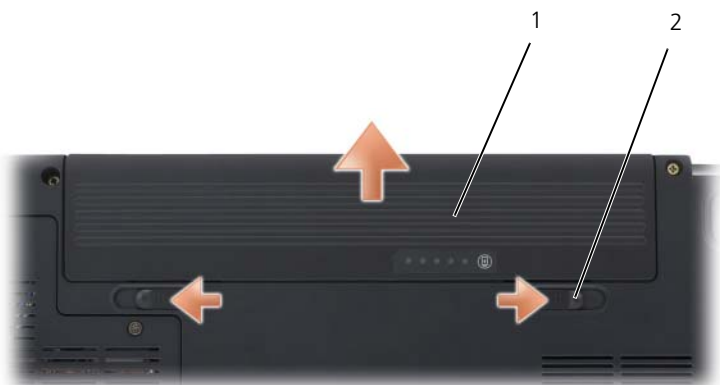
1 バッテリー 2 バッテリーリリーススラッチ (2)
